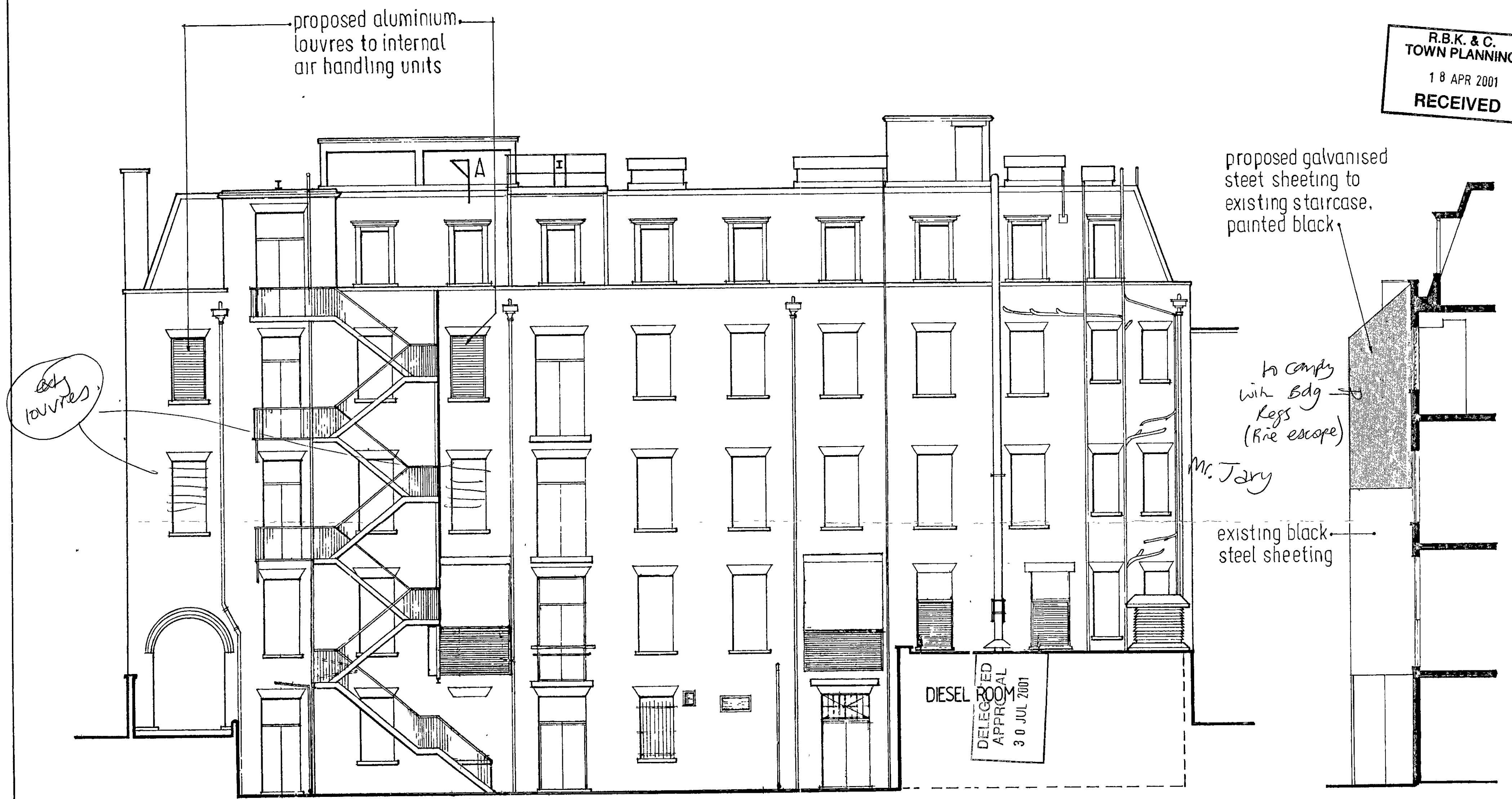
SECTION A-A
