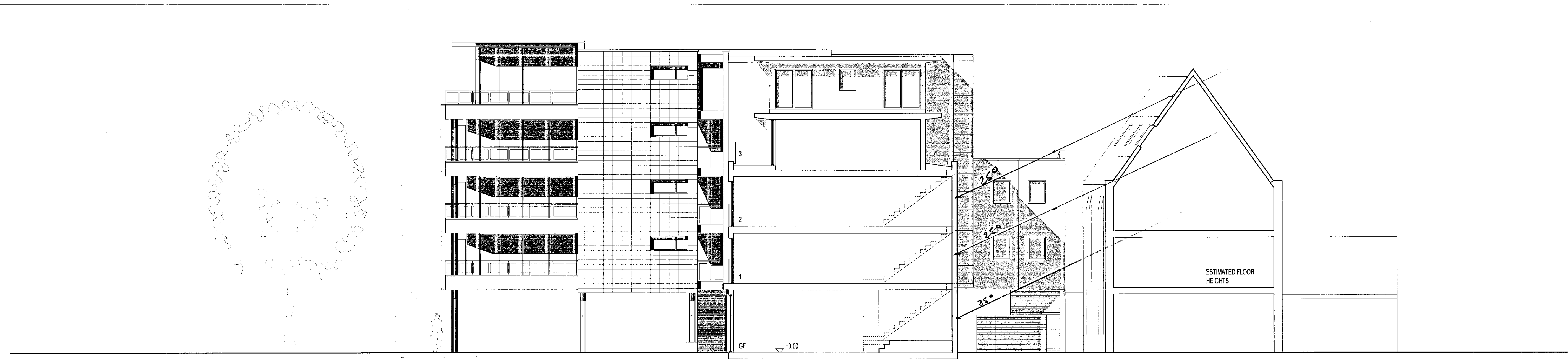
SECTION A-A
